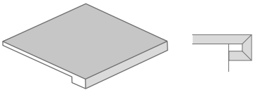
Peldaño Doble Gradone Fango Bianco 30x90 cm. 11 13/16 "x35 7/16 " P3090
